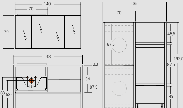
★ Quote di installazione consigliate Assembly dimensions recommended
